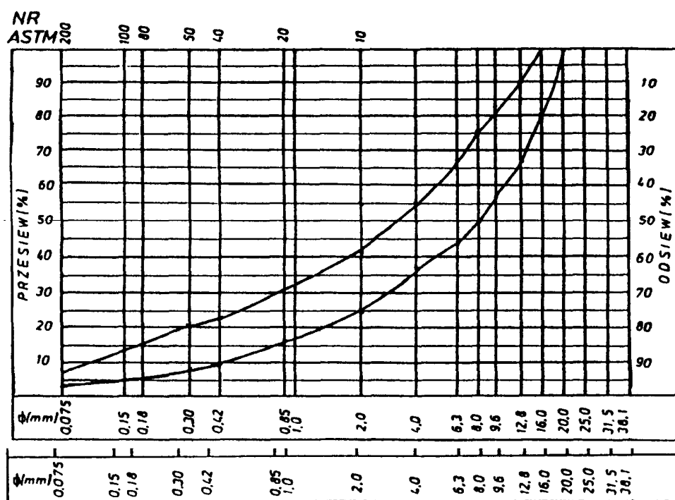
wzmacniającej z betonu asfaltowego dla KR 3-6
