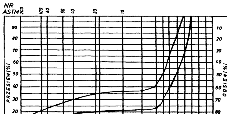
Rys. 5. Krzywe graniczne uziarnienia mieszanki mineralnej 0÷20 mm o nieciągłym uziarnieniu do warstwy ścieralnej z betonu asfaltowego dla KR 3-6
