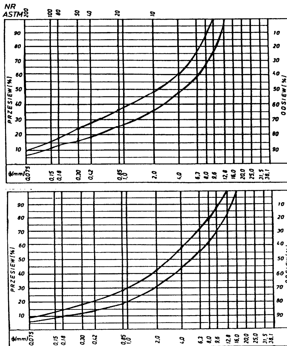
Rys. 6. Krzywe graniczne uziarnienia mieszanki mineralnej 0÷16 mm do warstwy ścieralnej z betonu asfaltowego dla KR 3-6
