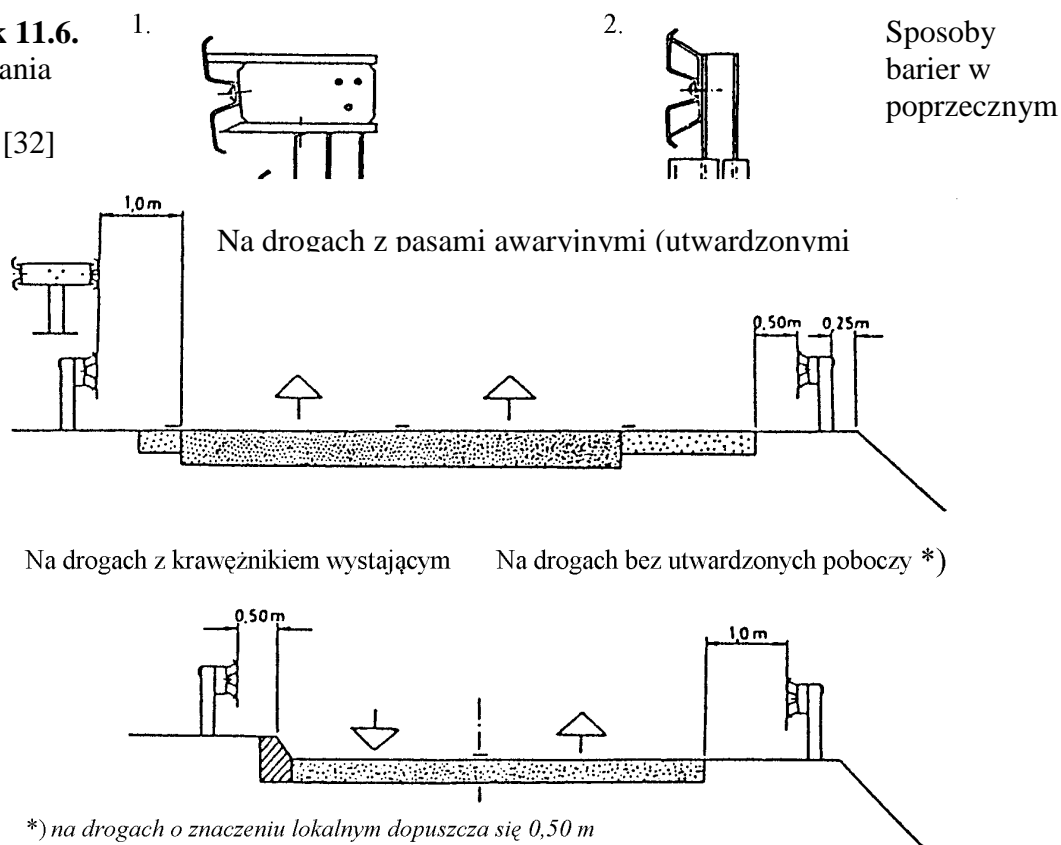
Załącznik 11.7. Zasady stosowania barier ochronnych stalowych na odcinkach dróg (wyciąg z WSDBO)
