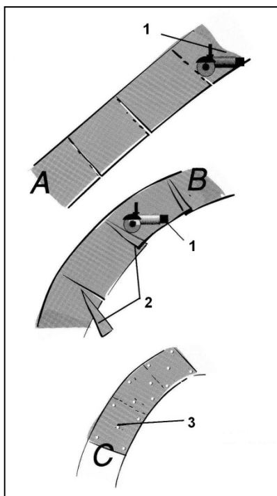
Rys. 4. Układanie siatki na łuku poziomym A - Nacięcie siatki od wewnętrznej krawędzi łuku B - Uformowanie łuku przez utworzenie zakładki w miejscach nacięć C - Przycięcie zakładki i przymocowanie siatki kołkami do podłoża 1 - piła, 2 - zakładki, 3 - kołki
